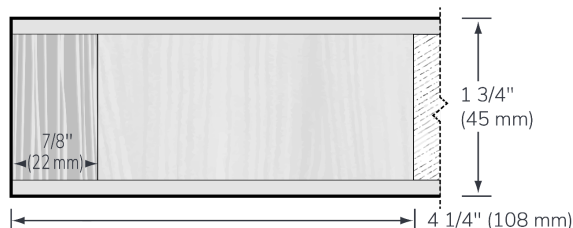
2 COUPE DES BATTANTS
